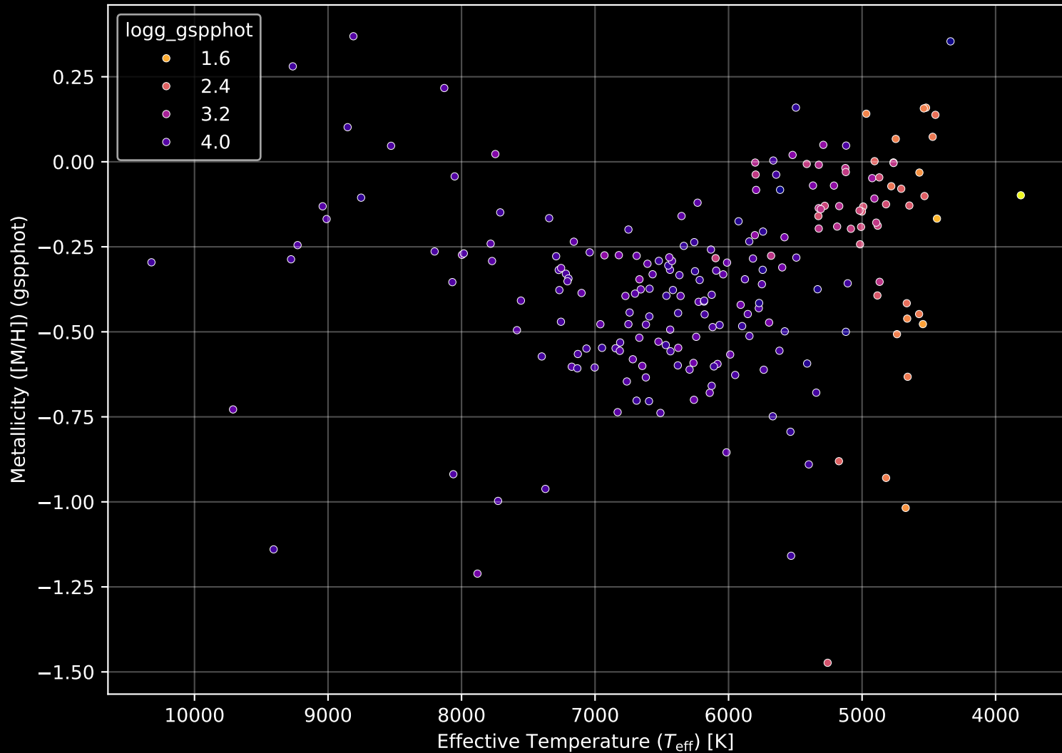
GALAH DR4 Field: [9468] Stellar Population Parameters (n= 215)
