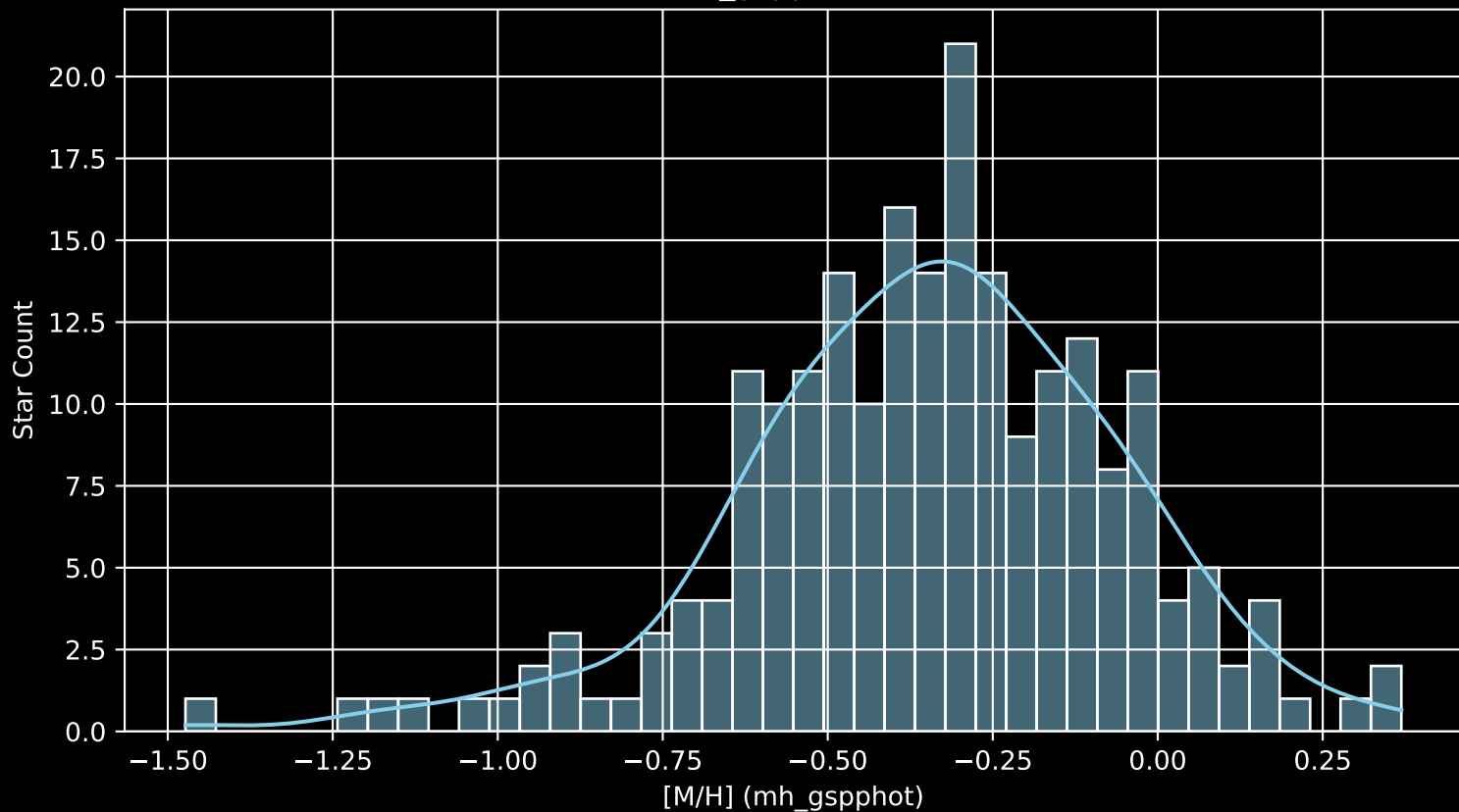
GALAH DR4 Field: [9468] [M/H] (mh_gspphot) (n= 215)
