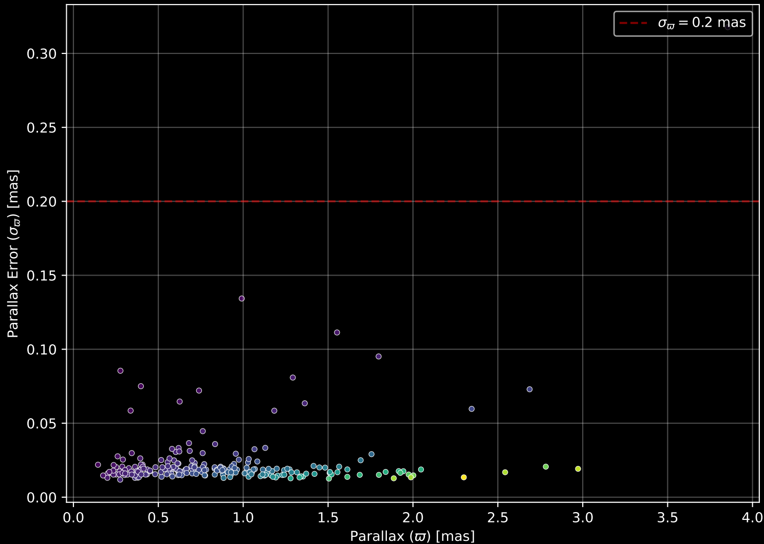
GALAH DR4 Field: [9468] Parallax Quality (n= 215)
