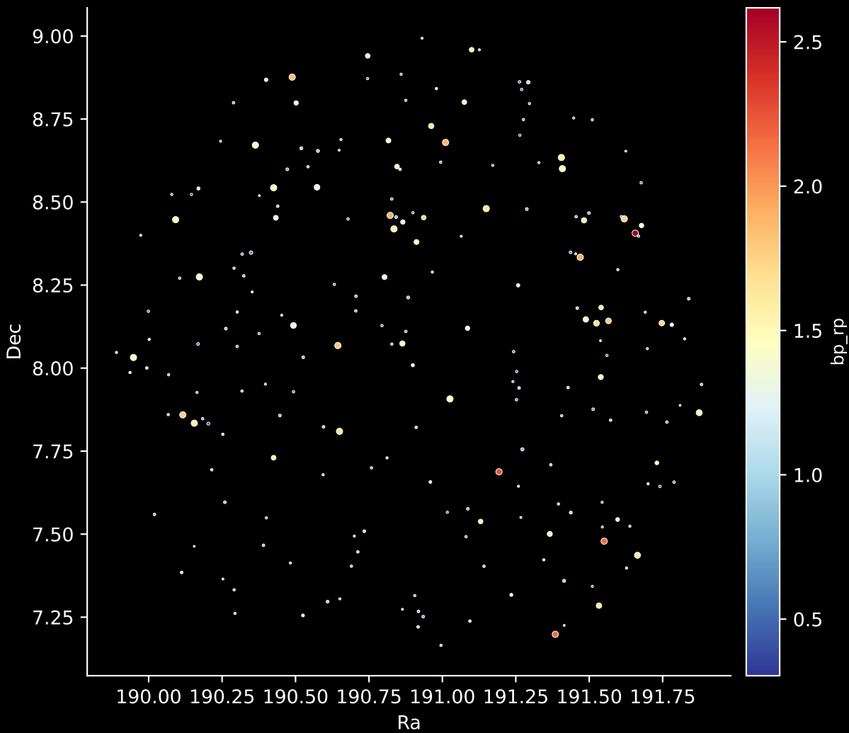
GALAH DR4 Field: [9468] Stars: 215
